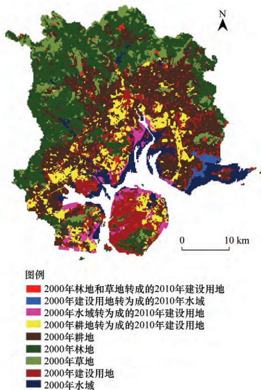
图 1 2000—2010 年间厦门市土地利用变化 Fig.1 Land-use change from 2000 to 2010 in Xiamen city
