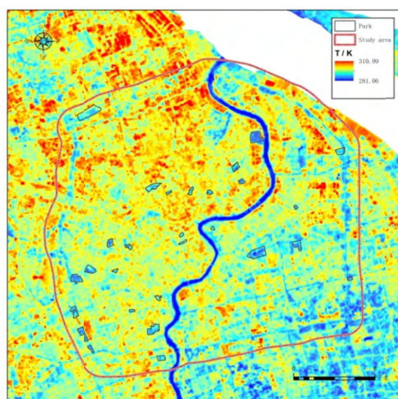
图 2 亮度温度空间分布
