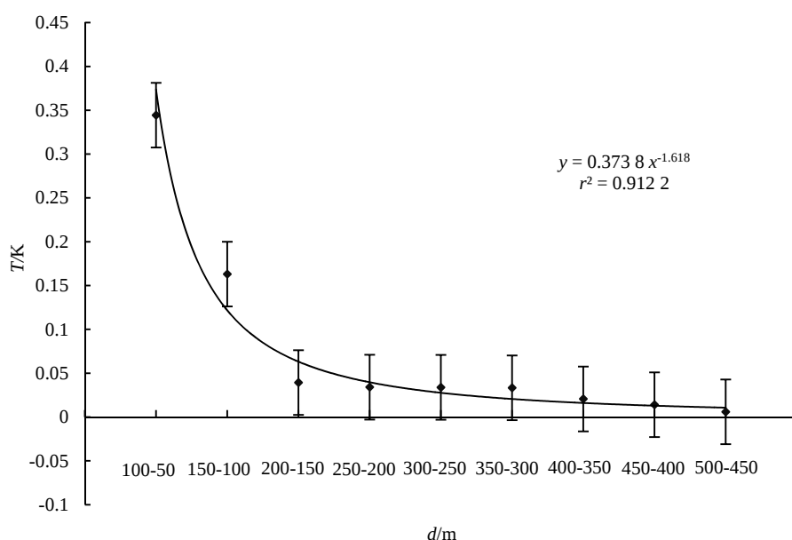
图5 绿地公园及周边降温幅度随距离的变化
