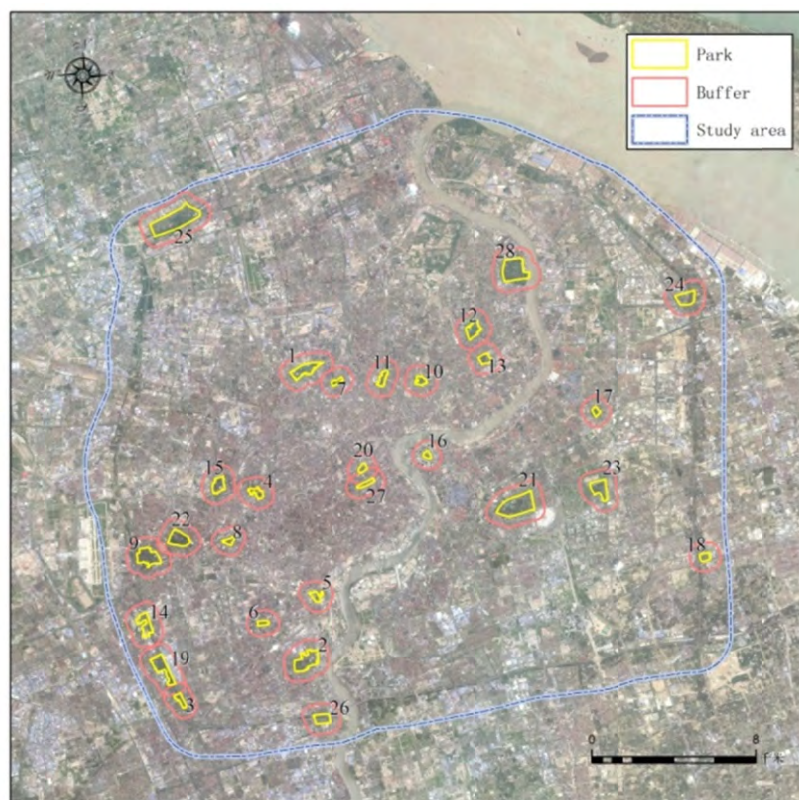
图 1 绿地公园位置分布
