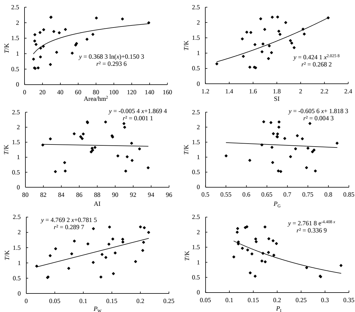
图7 绿地公园格局与降温幅度之间的关系
