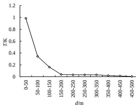
图6 绿地公园对周围环境降温幅度量化统计
