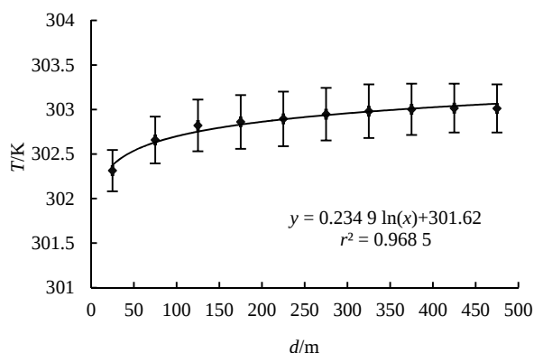
图4 绿地公园及周边温度随距离的变化
