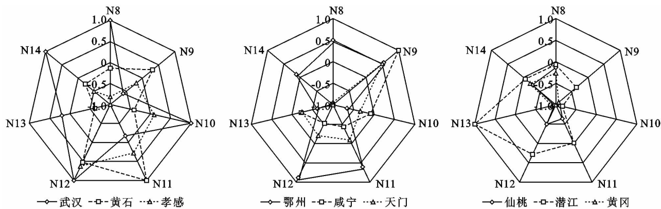
图 2 武汉城市圈土地碳汇适宜性评价示意图
