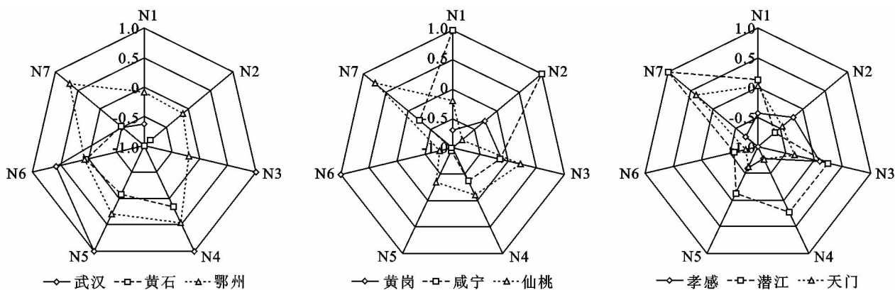
图 1 武汉城市圈土地碳源适宜性评价示意图
