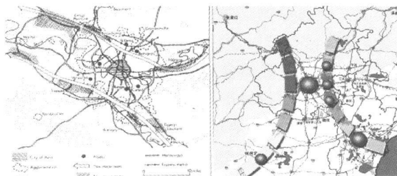
图 1 法国巴黎 1965 年规划与 2003 年北京空间发展战略比较
