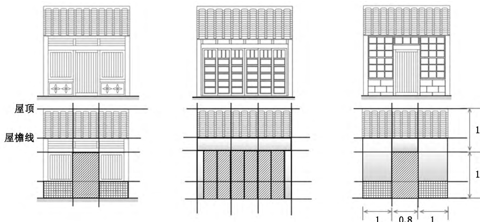
图2 总爷老街之清代建筑立面比例关系图
