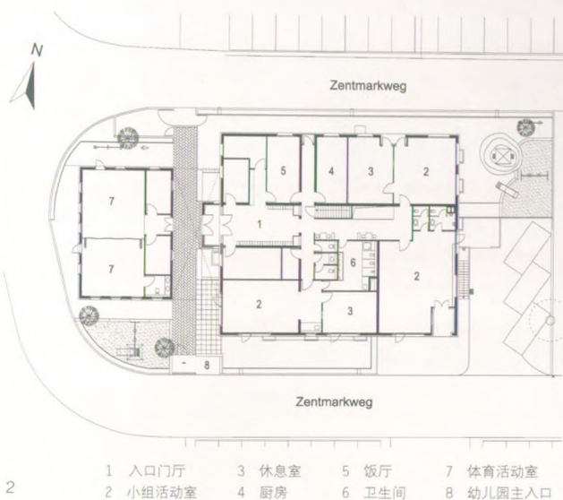
1 入口门厅 3 休息室 5 饭厅 7 体育活动室 2 小组活动室 4 厨房 6 卫生间 8 幼儿园主入口
